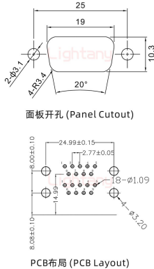
PCB布局 (PCB Layout)
