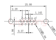
PCB布局 (PCB Layout)
