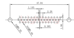
PCB布局 (PCB Layout)
